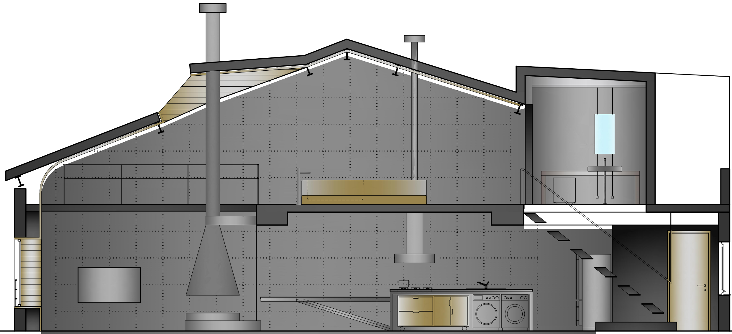
A-A SECTION
